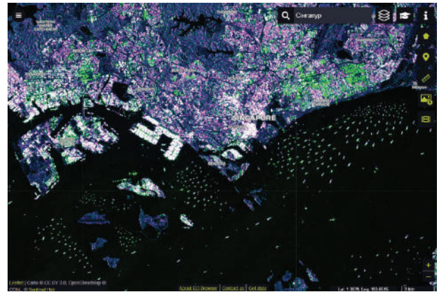
Sentinel-1 SAR-urban
