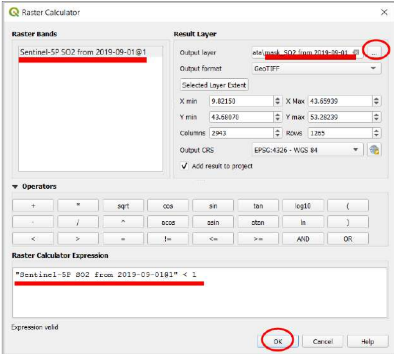
Рис. 2. 133. Створення маски хмар
