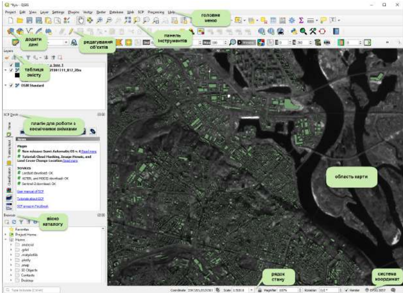
Рис. 1. 46. Інтерфейс робочого вікна проекту QGIS
