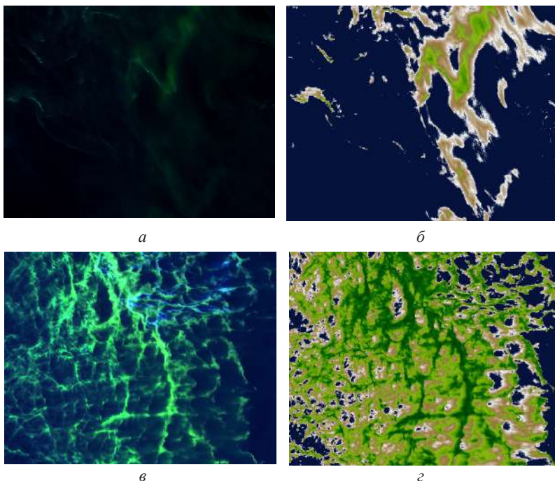
Рис. 2. 88. Динаміка поширення «цвітіння» води Київського водосховища на космічних знімках ( а – 6.08.2016 і б – 9.08.2016) та тематичних картах розподілу синьо-зелених водоростей отриманих на основі значень вегетаційного індексу ( б – 6.08.2016 і г – 9.08.2016)
