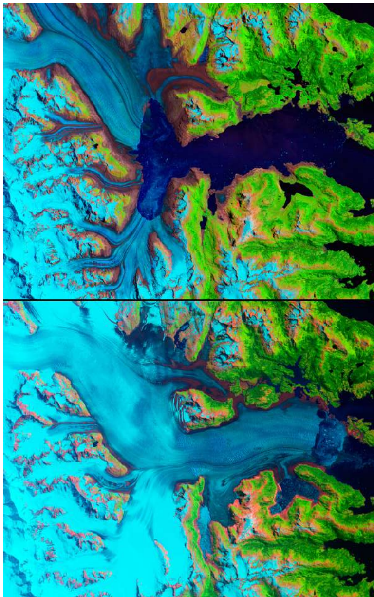
Рис. 4.7. Динаміка танення льодовика Колумбія на космічних знімках Landsat: a — 1980 р.; б — 2015 р. [7]
