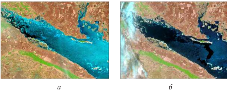
Рис. 4.22. Зображення льодових явищ на Кременчуцькому водосховищі, отримане супутником Sentinel-2: а — станом на 4 березня 2017 р.; б — станом на 11 березня 2017 р. [18]
