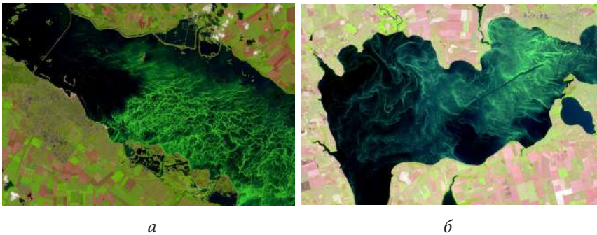
Рис. 4.11. Зображення явища «цвітіння води» супутником Sentinel-2 на прикладі: а — Кременчуцького водосховища, отримане 22 серпня 2015 року; б — Каховського водосховища, отримане 10 серпня 2016 року [7]
